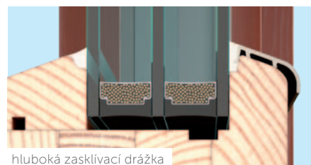
hluboká zasklívací drážka
