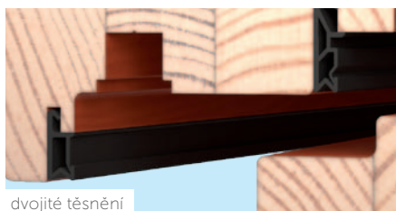
dvojitě těsnění
